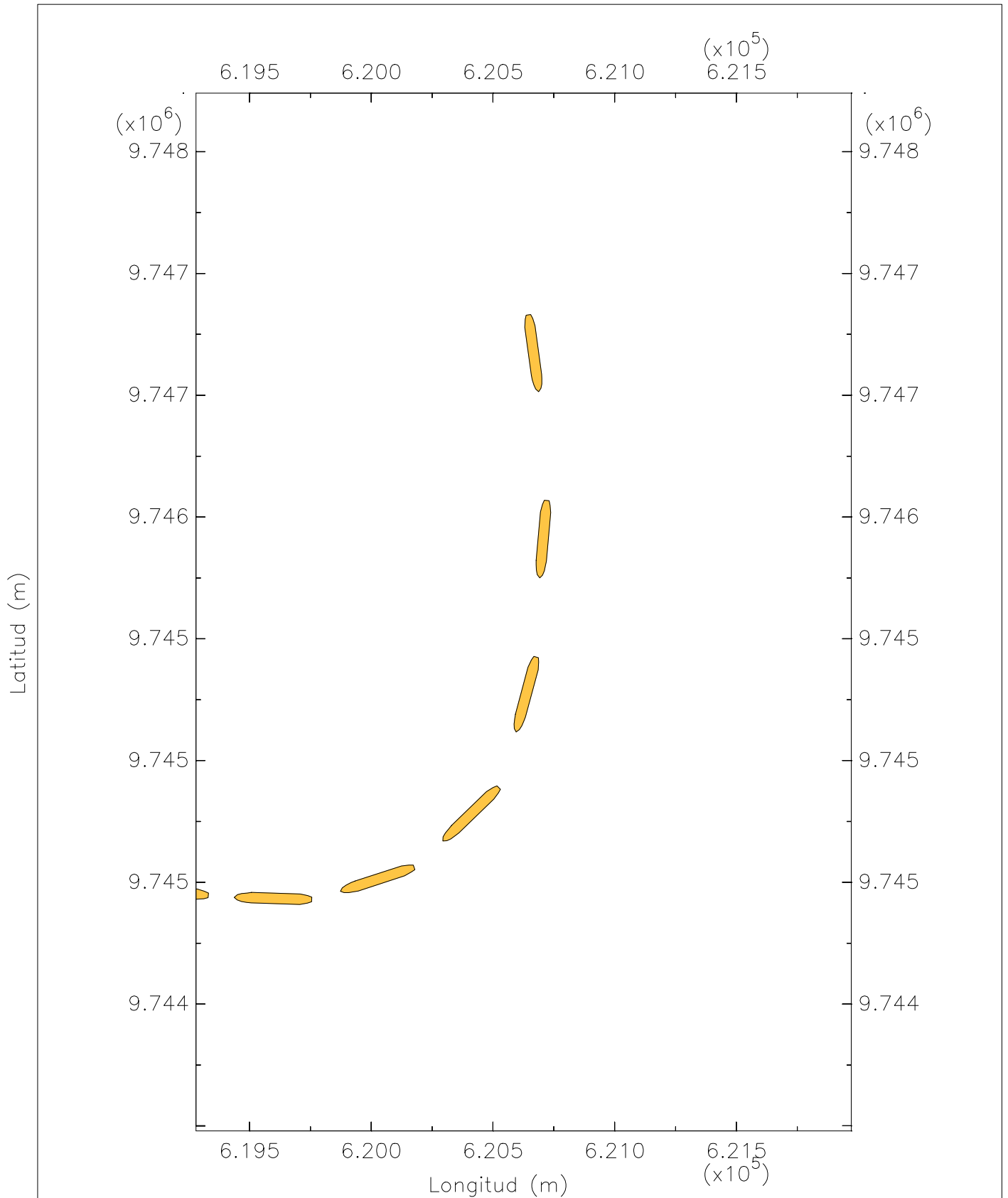
Z3T1 Trayectoria del barco portacontenedores en reflujos
