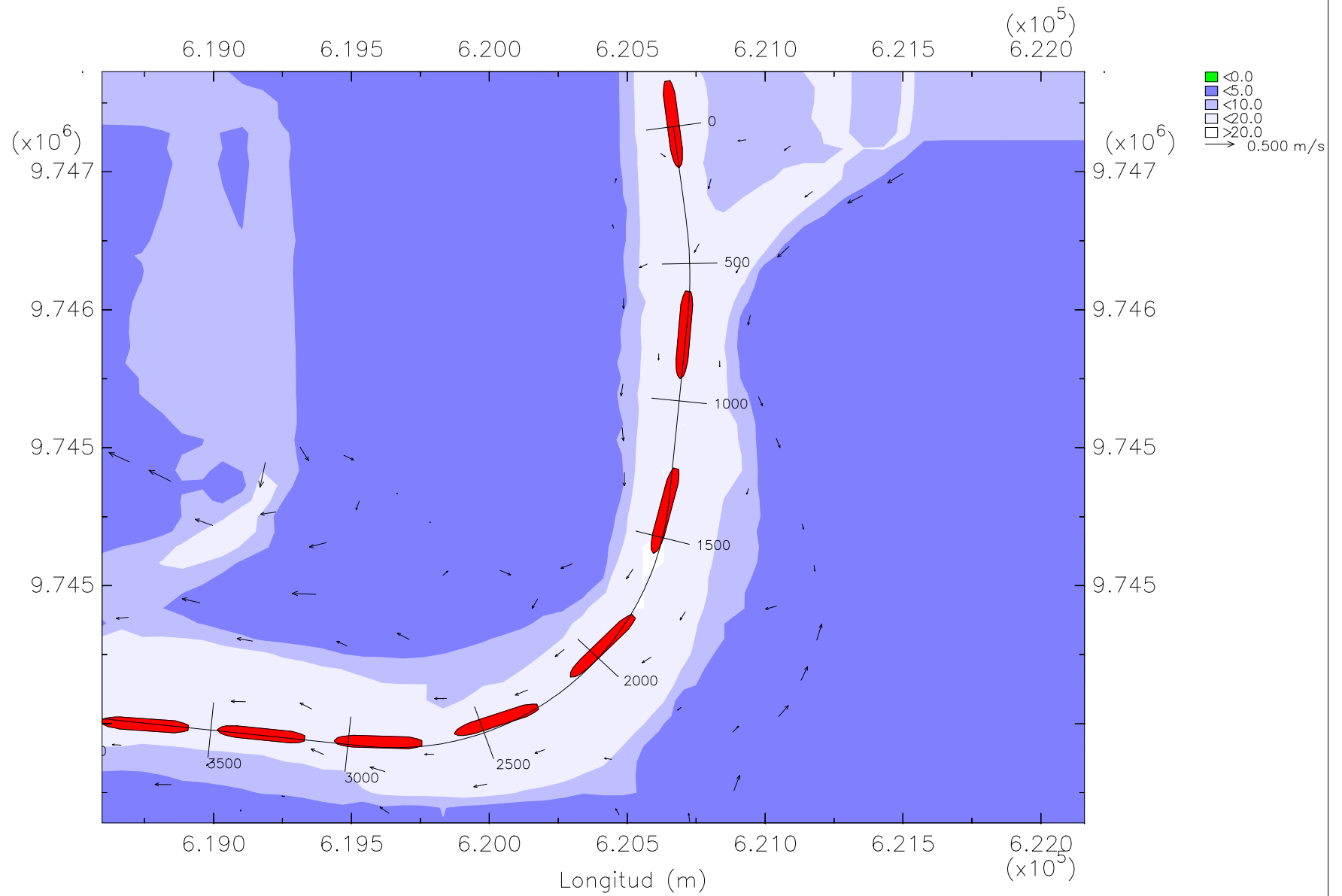
Z3T1 Trayectoria del barco portacontenedores post-panamax y corriente en reflujos
