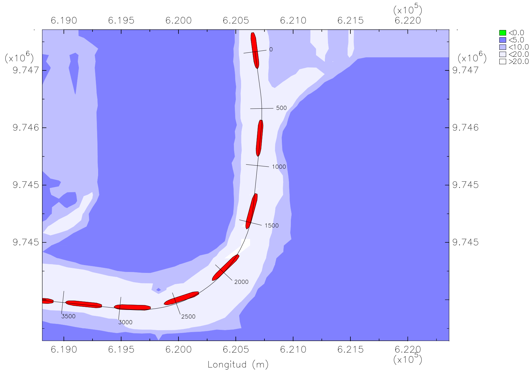
Z3T1 Trayectoria del barco portacontenedores post-panamax en reflujo
